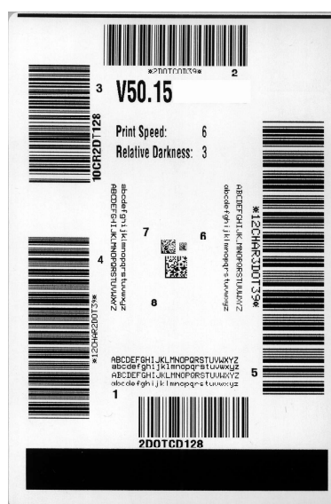
Abbildung 19 • Beispiel Testetikett für Schwärzung und Geschwindigkeit
