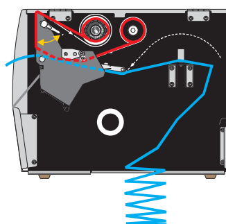
Unterer Eingabeschacht
