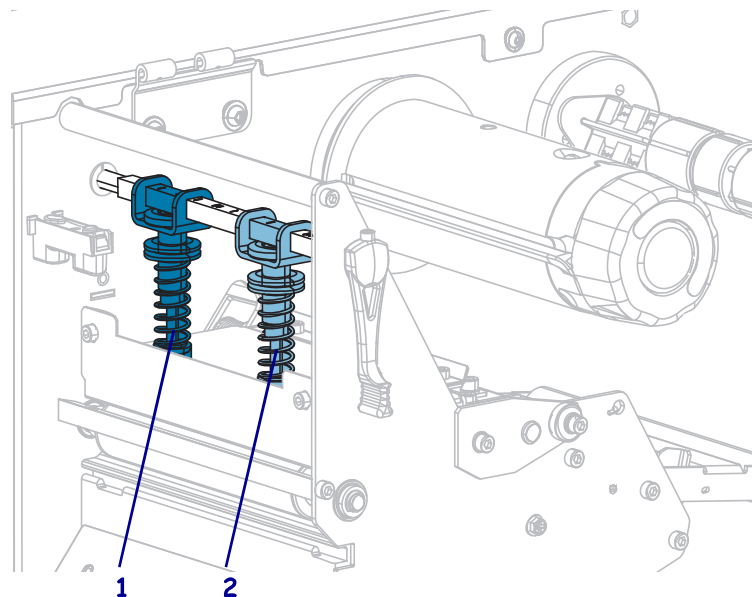
Abbildung 17 • Druckkopfdruk-Umschalter
