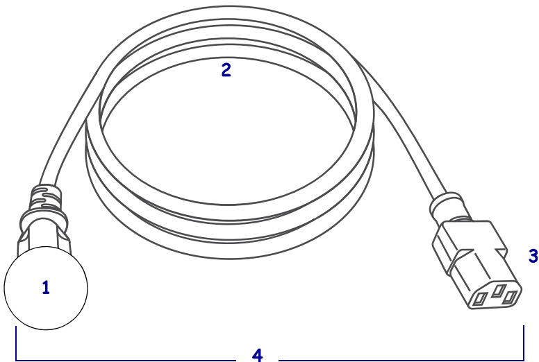
Abbildung 24 • Netzkabelspezifikationen
