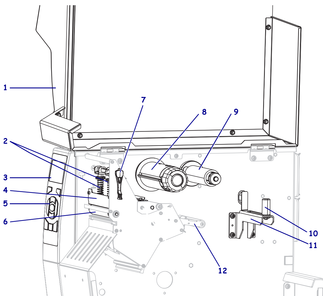
Abbildung 1 • Drucker-Komponenten
