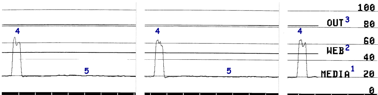
Abbildung 21 • Mediensensorprofil (Medien mit Zwischenräumen/Lücken)
