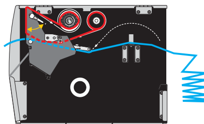
Hinterer Eingabeschacht
