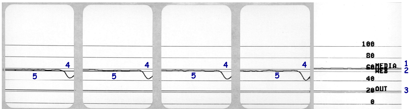
Abbildung 22 • Mediensensorprofil (Medien mit schwarzen Markierungen)
