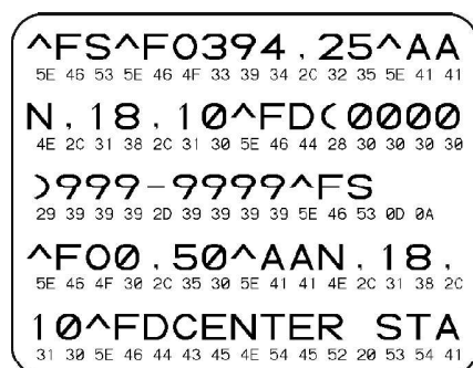
Abbildung 6 Beispielticket des Kommunikationsdiagnosemodus
