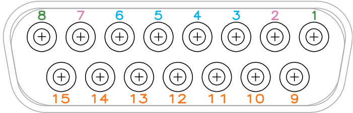
Abbildung 10 Externe Pol-Belegungen
