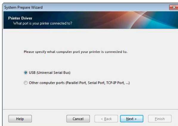
Abbildung 15 Systemvorbereitungsassistent
