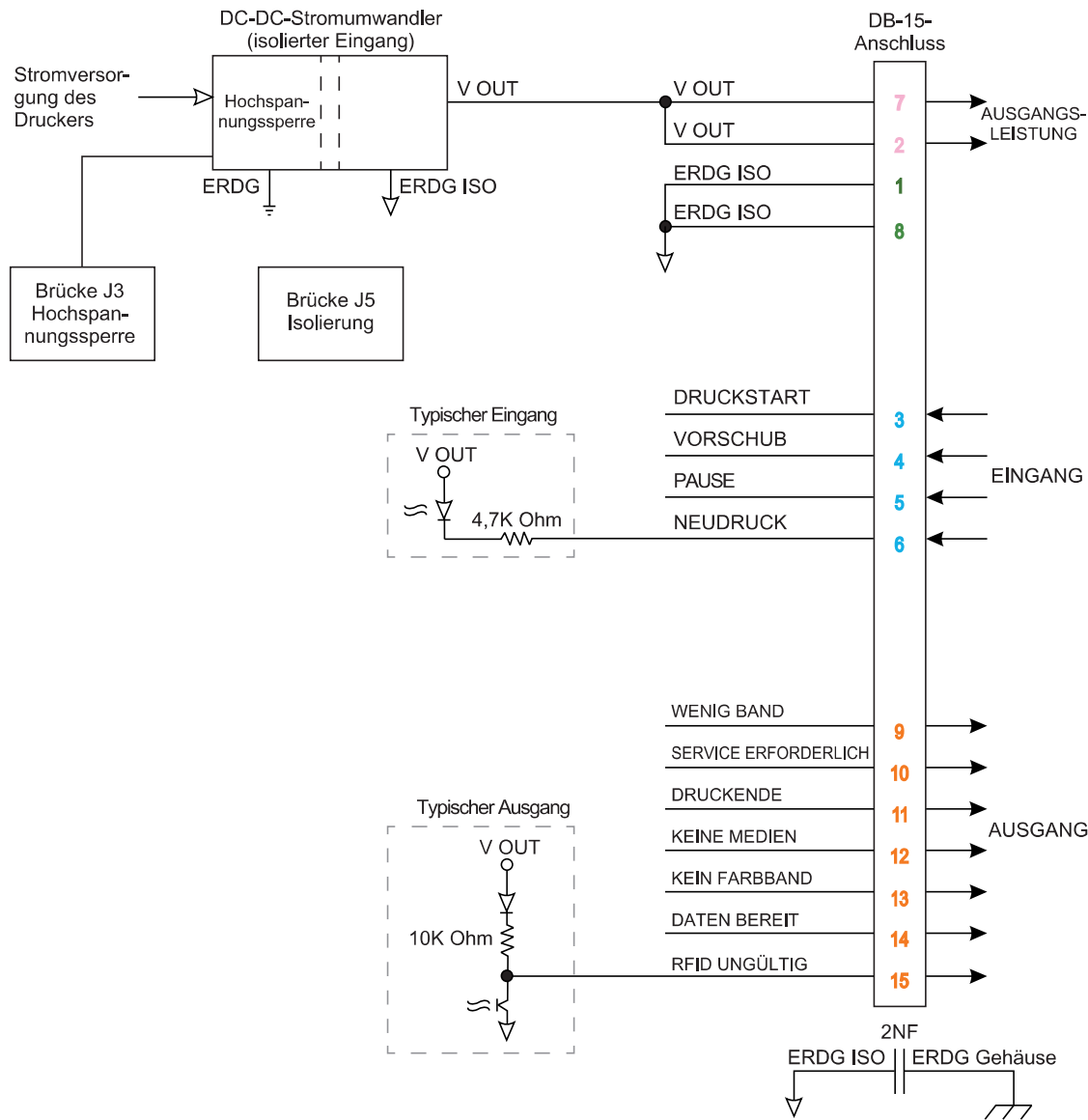
Abbildung 10 Externe Pol-Belegungen
