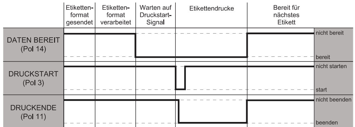
Abbildung 12 Applikator-Signale (Modus 2)
