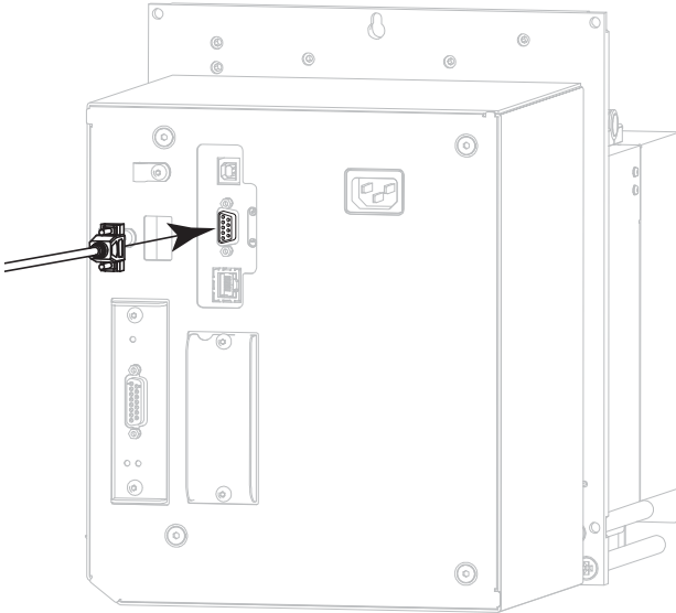
Serieller Anschluss
