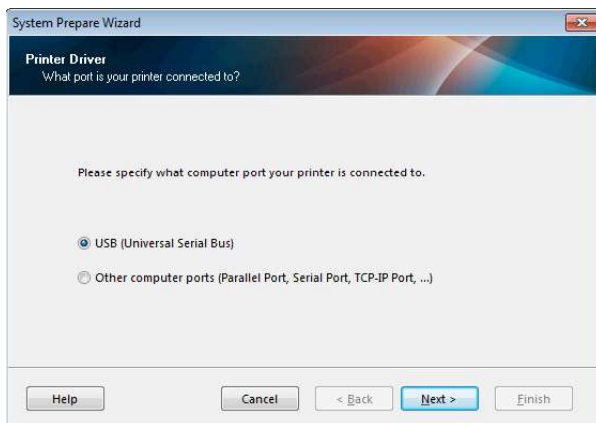
Abbildung 17 Systemvorbereitungsassistent
