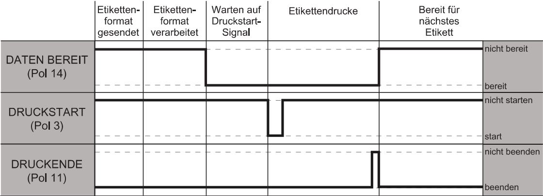
Abbildung 14 Applikator-Signale (Modus 4)
