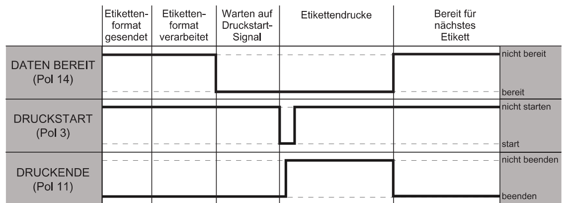
Abbildung 13 Applikator-Signale (Modus 3)
