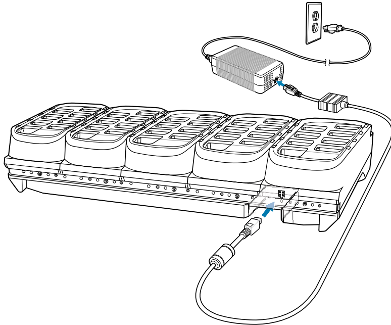
Abbildung 13 Einrichten des Vierzigfach-Akkuladegeräts
