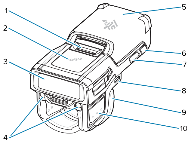
Abbildung 2 Doppelauslöser-Konfiguration – Draufsicht
