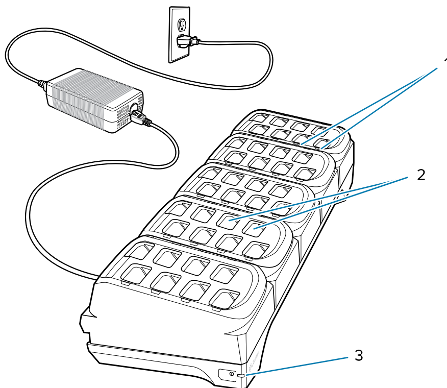
Abbildung 12 Vierzigfach-Akkuladegerät
