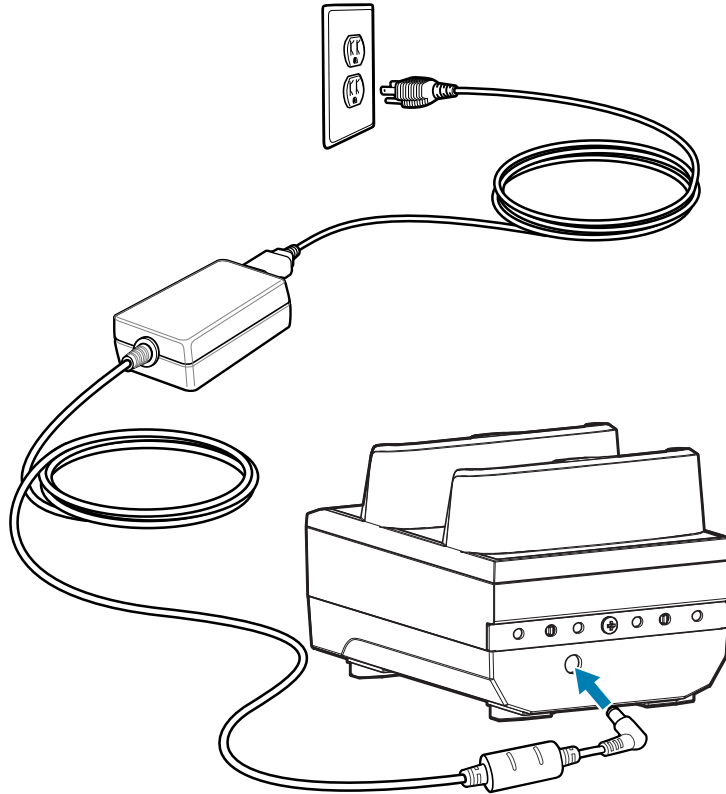
Abbildung 7 Einrichten der Vierfach-Ladestation
