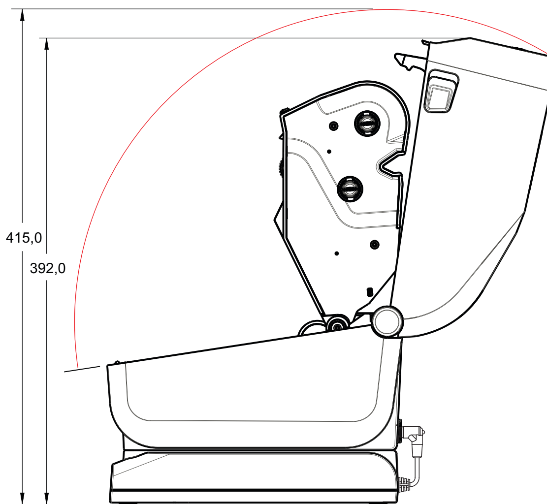
Drucker mit Netzteil-Basisstation
