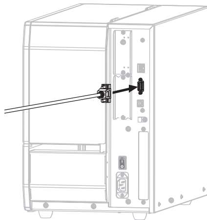
Serieller Anschluss
