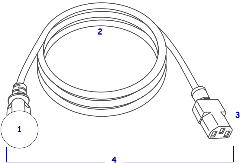
Abbildung 25 • Netzkabelspezifikationen
