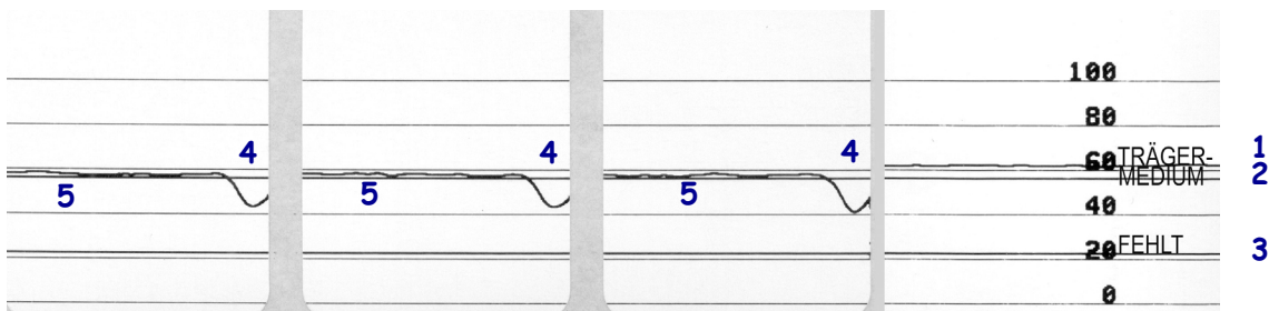
Abbildung 22 • Sensorprofil (Medienabschnitt)
