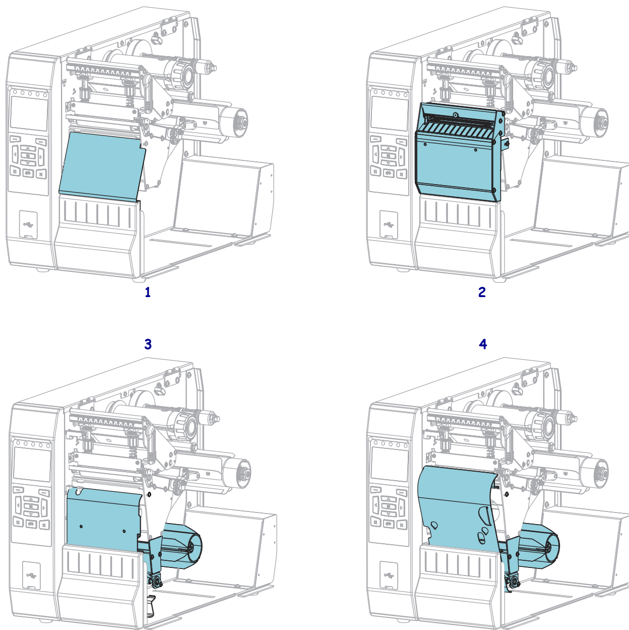
Abbildung 2 • Druckeroptionen
