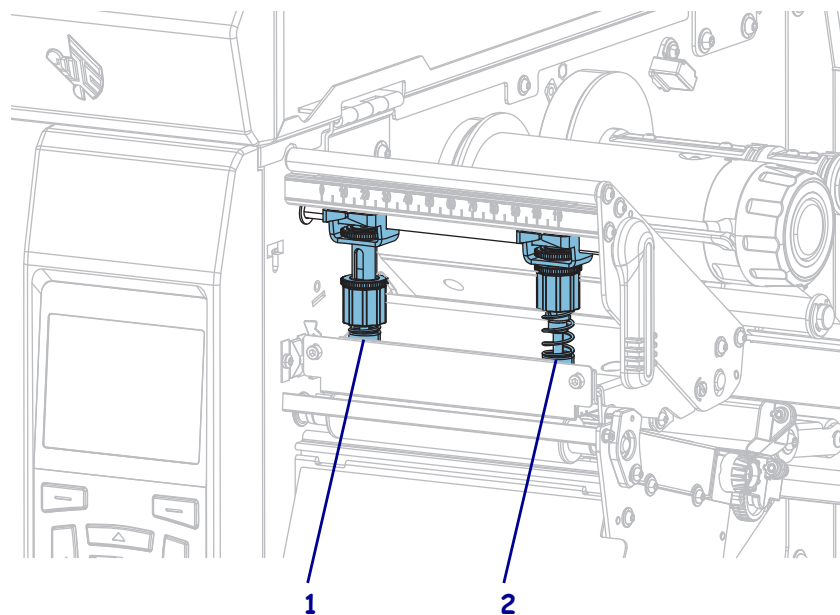
Abbildung 17 • Druckkopfdruck-Umschalter
