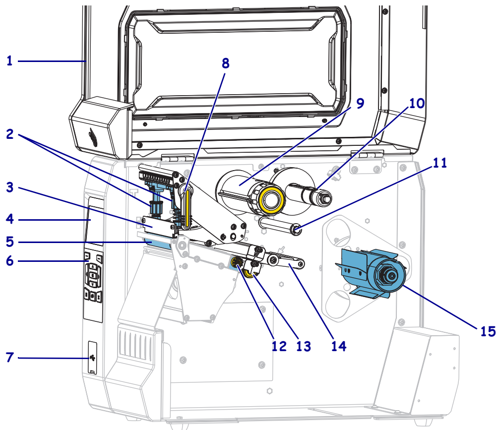
Abbildung 1 • Druckerkomponenten
