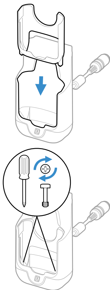
CTX-VD-CNV
