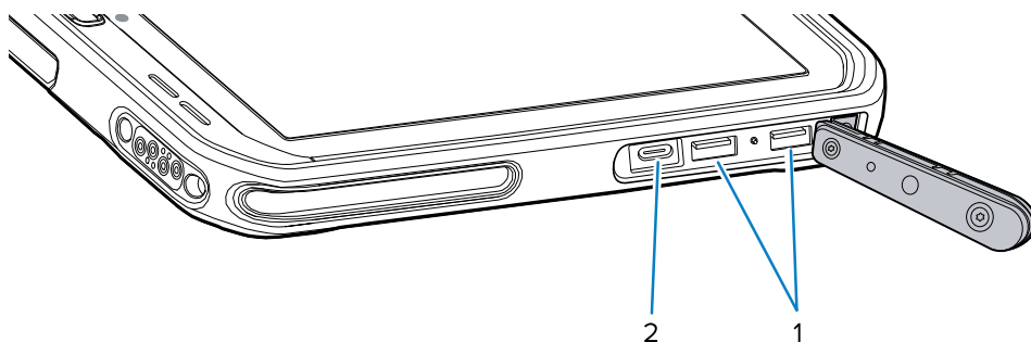
Abbildung 2 USB-Anschlüsse
