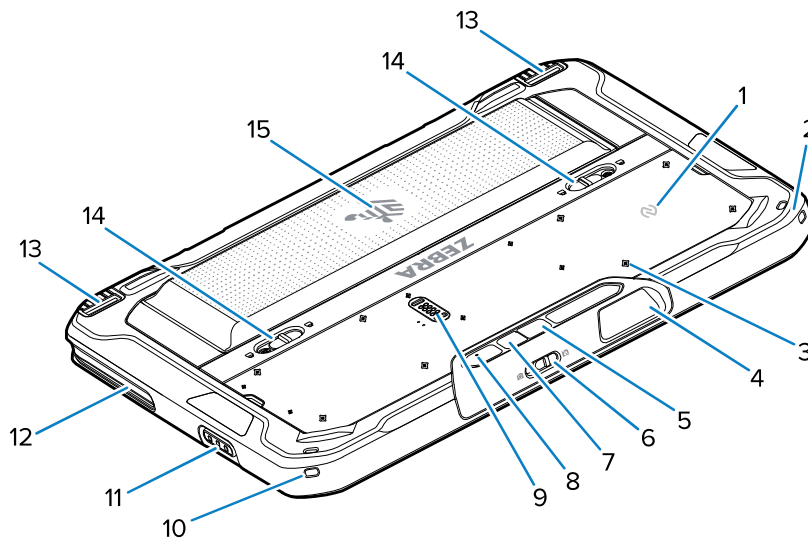
Abbildung 3 ET6x – Rückansicht
