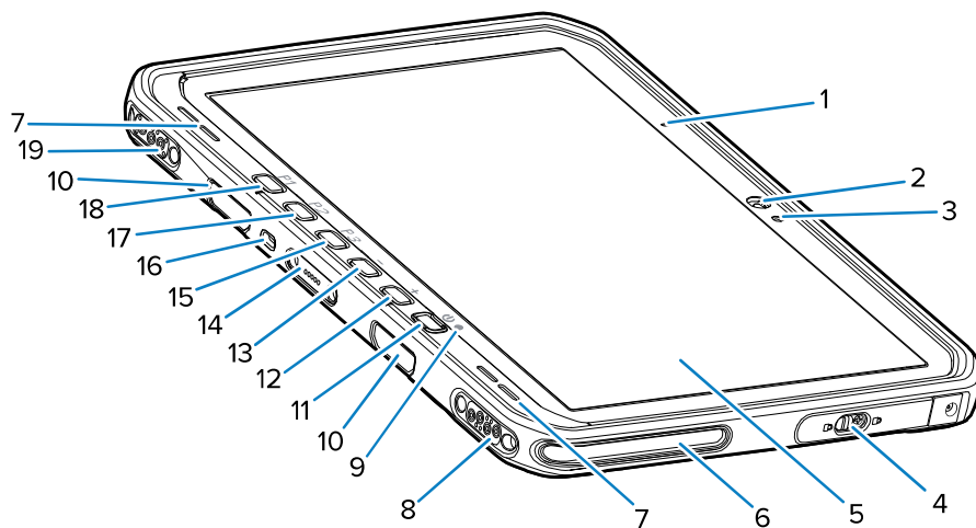
Abbildung 1 ET6x – Frontansicht
